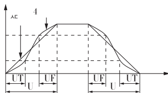
图 F 1 - 3 直线线加减速示意图
