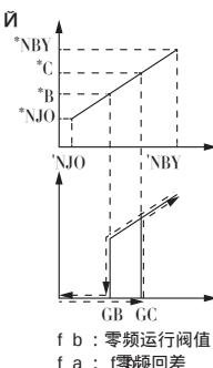
图 F6-1 零频功能示意图
