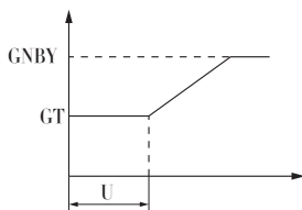
图 F1 - 1 启动频率示意图
