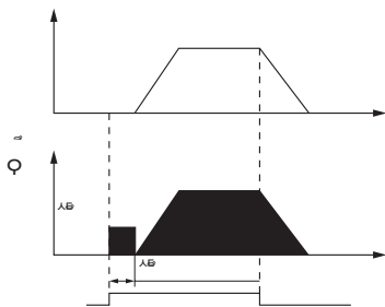
图 F1 - 2 启动直流制动示意图
