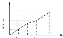
图 F5 - 2 用户设定 V/F 曲线示意图
