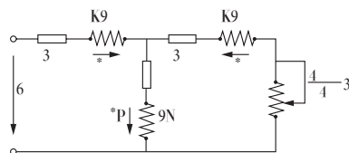
图 F 2 异步电机稳态等效电路图
