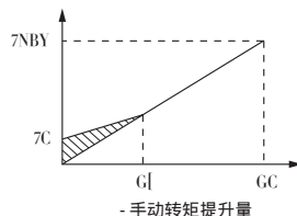
图 - 转矩提升示意图
