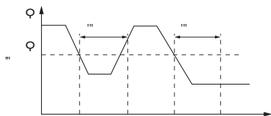
图 F A - 4 闭环反馈丢失检出时序图
