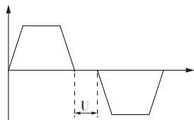
图 F 1 - 7 正反转死区时间示意图
