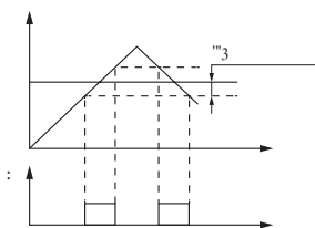
图 F 7 - 7 频率到达示意图
