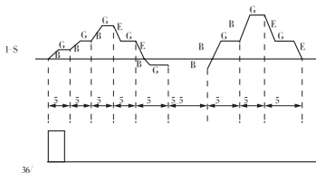
图 F 9 - 1 单循环后停机示意图
