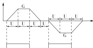
图 F 1 - 5 点动运行图
