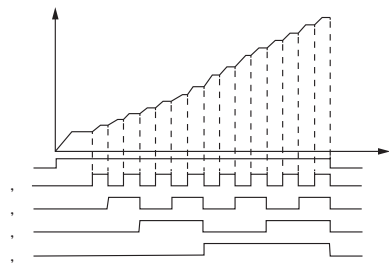
图 F 7 - 1 多段速运行示意图
