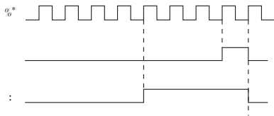
图 F 7 - 9 计数器复位设定和计数器检测设定示意图
