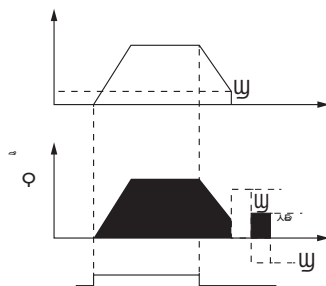
图 F 1 - 4 停机直流制动示意图
