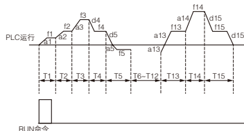
图 F9-1 PLC 单循环后停机示意图
