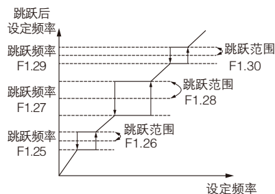
图 F1-6 跳跃频率示意图
