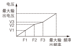
图 F5-2 用户设定 V/F 曲线示意图
