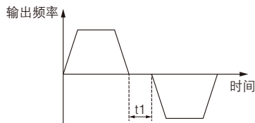
图 F1-7 正反转死区时间示意图
