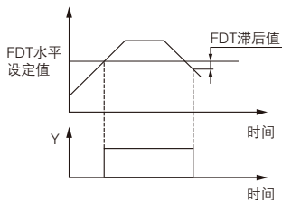
图 F7-8 频率水平检测示意图
