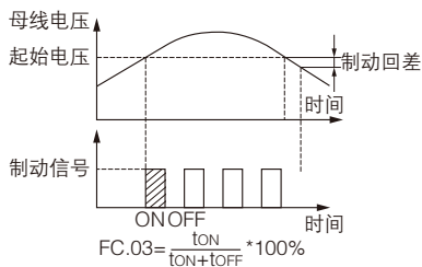
图 FC-1 能耗制动示意图
