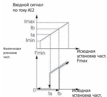
Рис. F6-1 Принципиальная схема функции нулевой частоты
