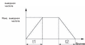
Рисунок F0-2. Время ускорения и замедления
