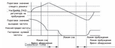
Рис. F8-5 Первый спящий режим
