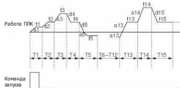
Рис.F9-2 Сохранение последнего этапа после одиночного цикла
