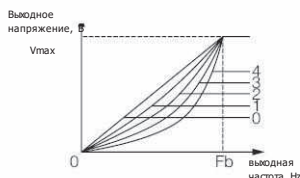
Vmax — максимальное выходное напряжение, Fb — максимальная выходная частота
