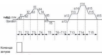
Рис. F9-1 Остановка после одного цикла ПЛК
