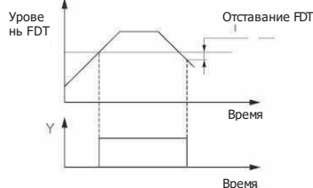
Рис. F7-8 Определение уровня частоты
