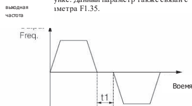
Рис. F1-7. Время перемещения вперед/назад и зона нечувствительности
