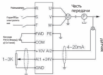
Рис. F8-1 Аналоговая система управления с обратной связью. ПИД-регулирование осуществляется следующим образом:
