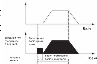
Рисунок 1-2. Торможение постоянным током на этапе запуска
