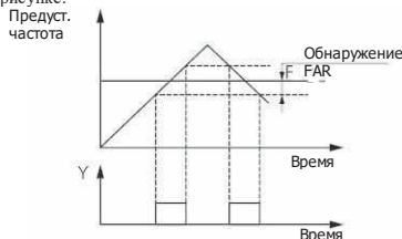
Рис. F7-7 Достижение частоты
