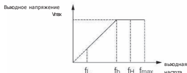
Рисунок F0-1. Напряжение и частота
