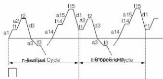
Команда запуска рис.г9-3 непрерывный цикл ПЛК
