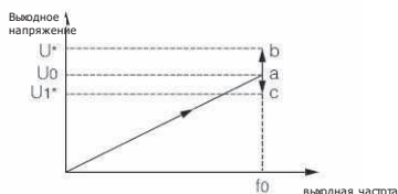
Рис. F5-4. Режим управления напряжением 0
