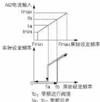
图 F6-1 零频功能示意图
