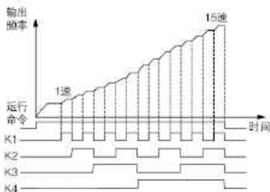
图 F7-1 多段速运行示意图
