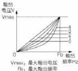
图 F5-1 V/F 曲线示意图
