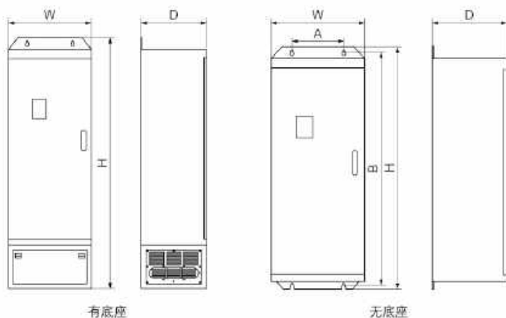
图A-3 160~350kW机型外形尺寸 (380V)
