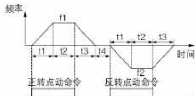
图 F1-5 点动运行图
