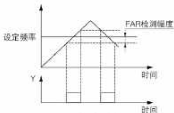
图 F7-7 频率到达示意图
