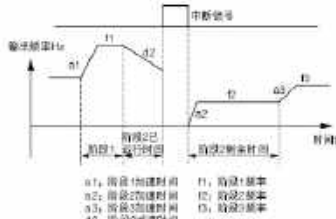
图 F9-4 PLC 启动方式 1
