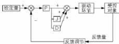
图 F8-2 PID 调节示意图
